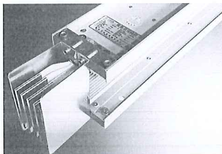
母线槽产品
