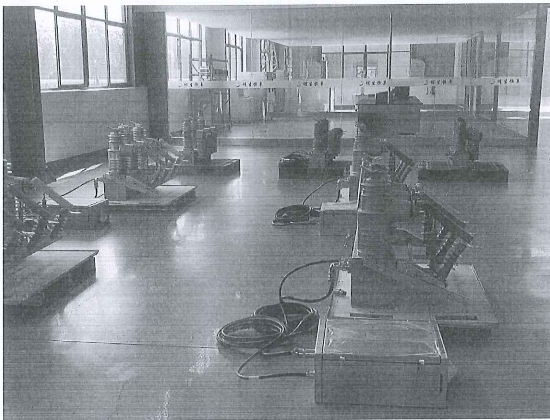
ZW32-12/630-20 一二次融合成套柱上断路器
