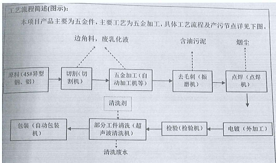
工艺流程图
