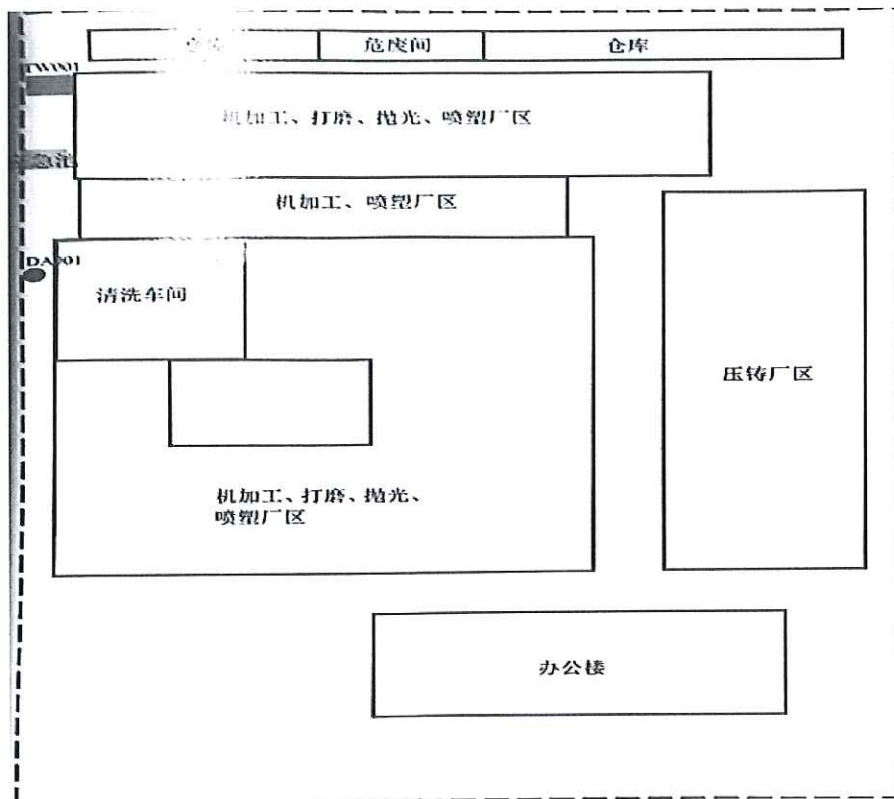
厂区布局图
