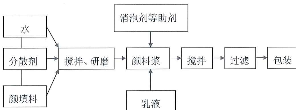
产品生产工艺流程图
