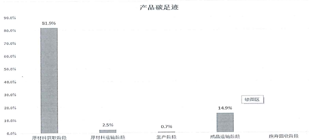
图 5.2-2 生命周期阶段碳排放分布图
