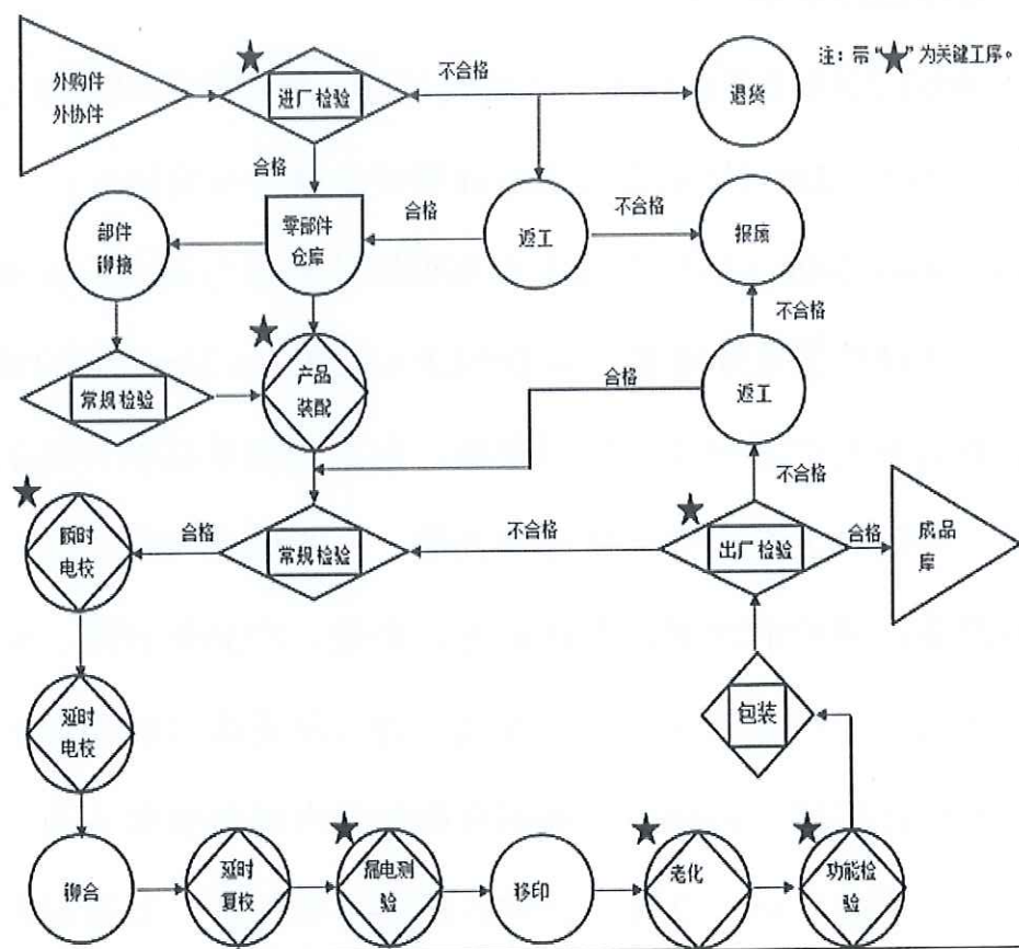
图 2.3 工艺流程图
