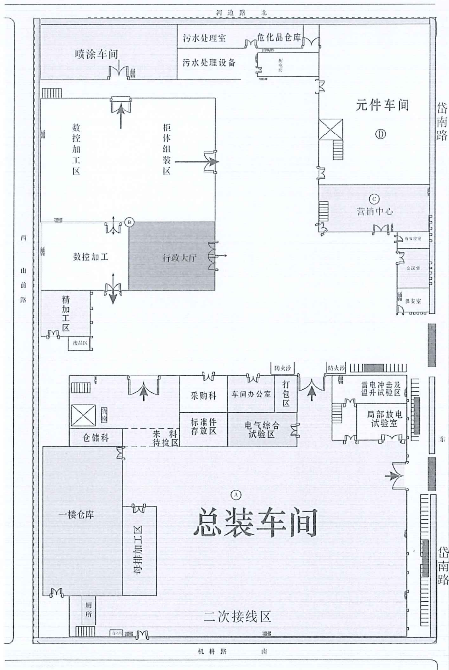
图 2.2 厂区布局图
