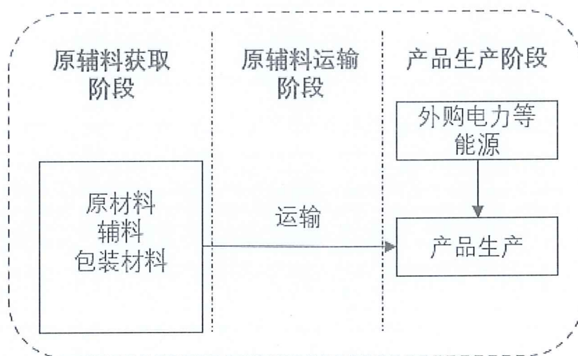
图 3.1 柱上开关产品碳足迹评价系统边界
