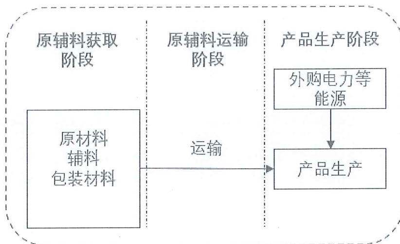
图 3.1 标准化配电变压器产品碳足迹评价系统边界
