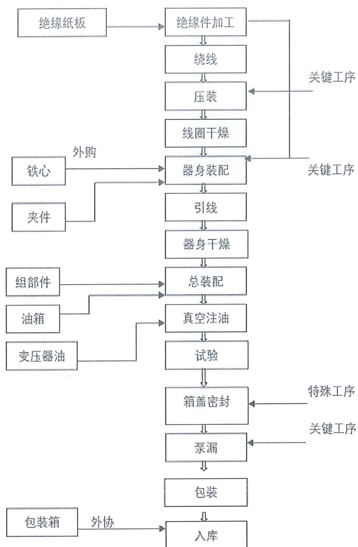
图 2.3 产品生产工艺流程图
